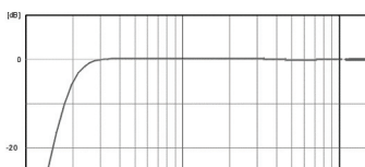
Illustration 6 : Filtre en plateau >6 kHz pour les fréquences supérieures à 6 kHz
